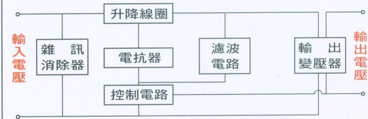
方塊圖
